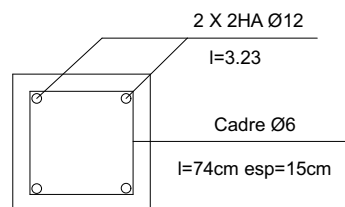
Details de ferrailage du Poteau
