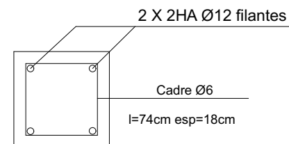
Details de ferrailage du chainage haut
