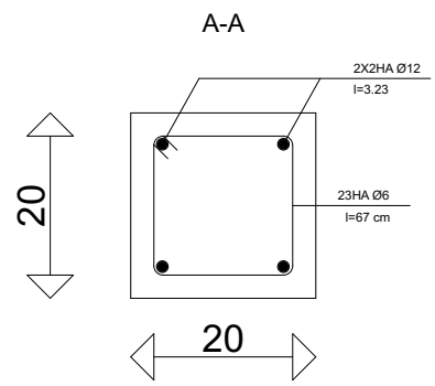
Details de ferrailage du poteau
