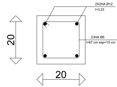
Details de ferrailage du chaînage horizontale
