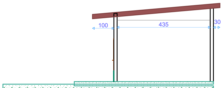
COUPE AA
